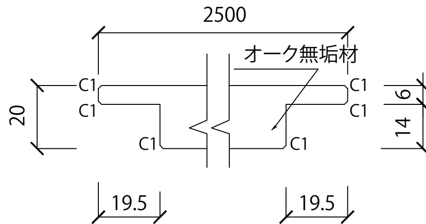
長手断面図
