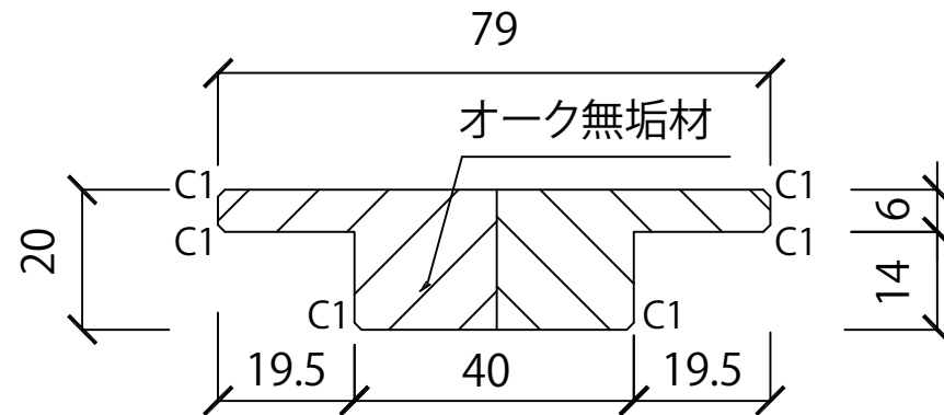
短手断面図
