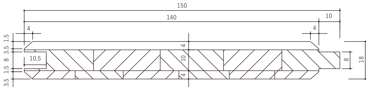
断面図
