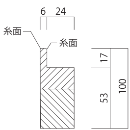
■断面図〔パイン・ウレタン着色塗装〕
