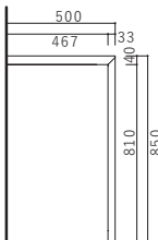
断面図
