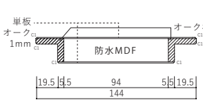
■断面図（オーク【複合】）
