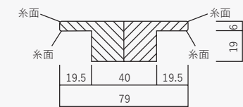
■断面図（ウレタン着色塗装）
