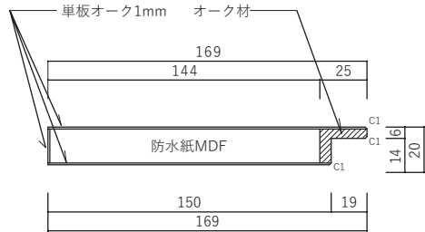
■断面図（オーク）
