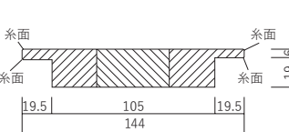
■断面図（パイン・ウレタン着色塗装）
