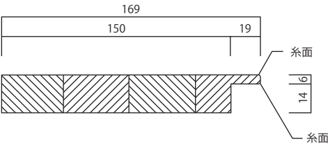
■断面図（パイン・ウレタン着色塗装）
