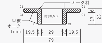
■断面図（オーク【複合】）
