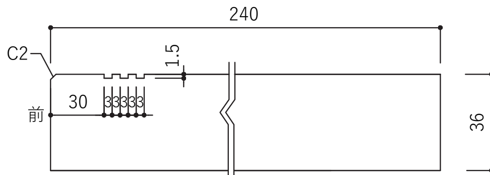
加工図
