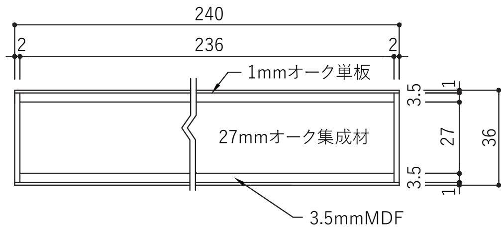
1000×240×36mm 断面図
