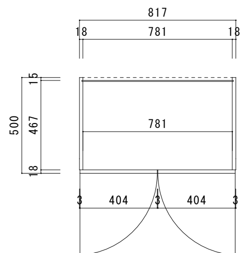
組立完成平面図
