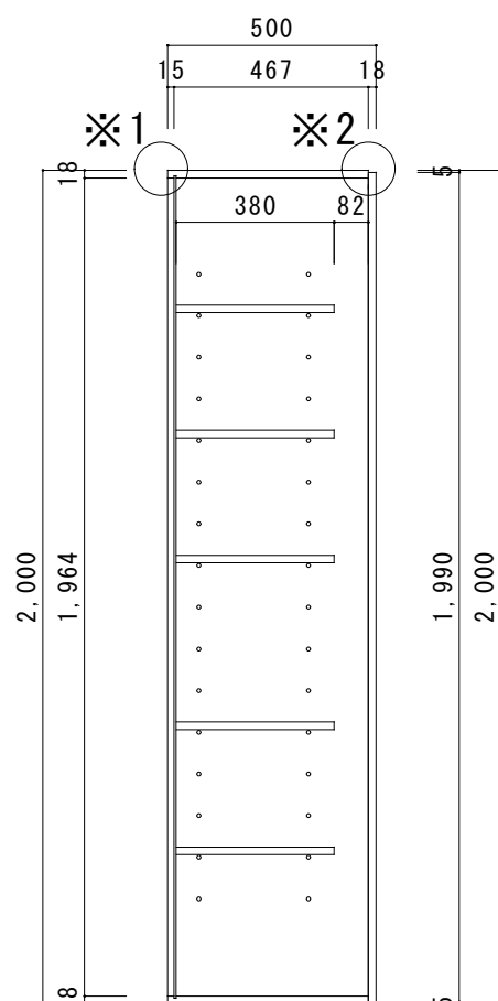
組立完成断面図
