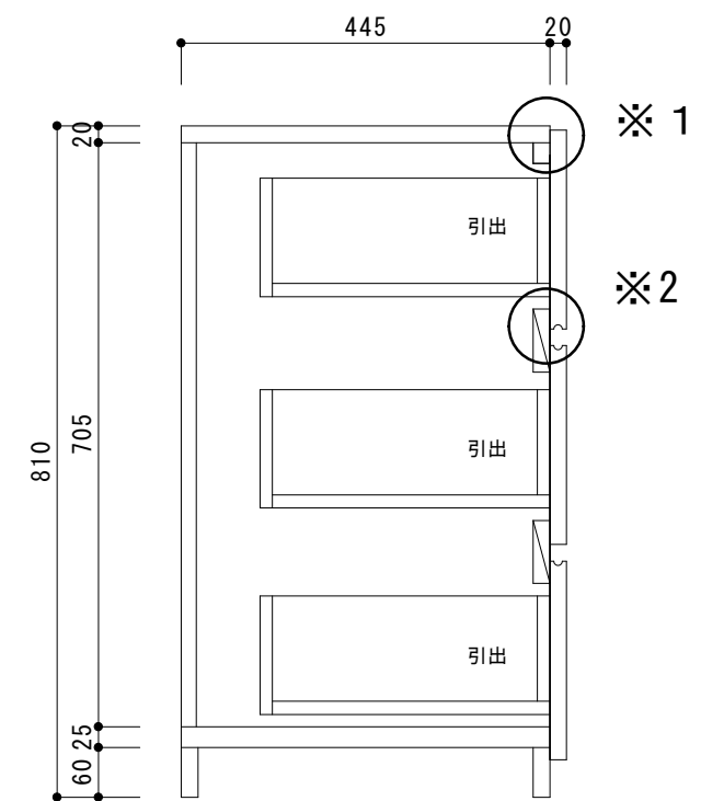
断面図(引出) B-B'
