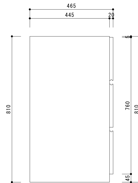
断面図(引出) A-A'
