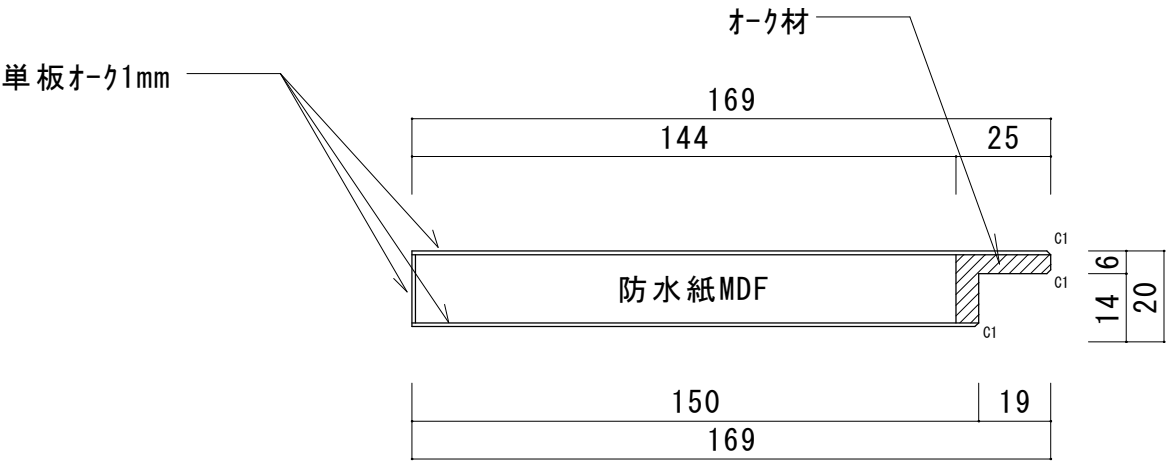
断面図
