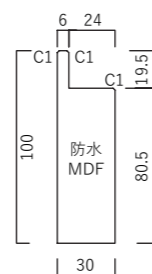
■断面図 (ウレタン着色塗装)
