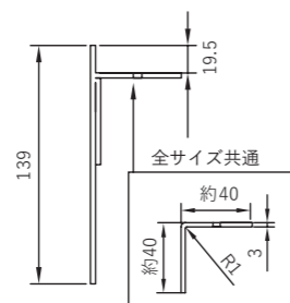
■断面図 (スチール)
