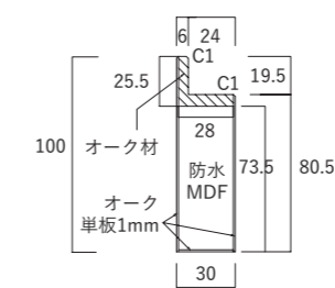
■断面図(オーク【複合】)
