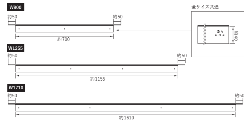
■平面図 (スチール)
