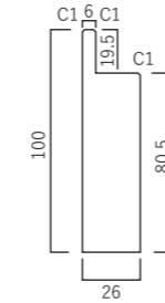
■断面図(オーク【無垢】)
