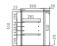
断面図
