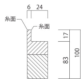
■断面図（パイン）
