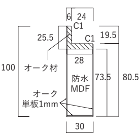
■断面図（オーク【複合】）
