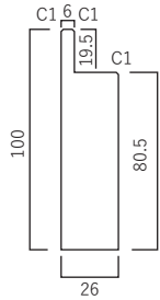
■断面図（オーク【無垢】）
